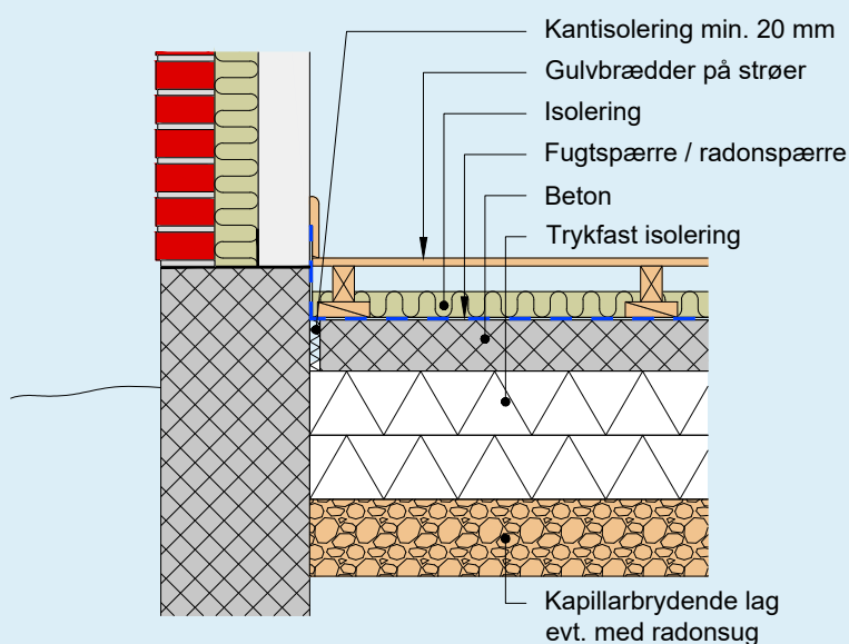
Nyt terrændæk
